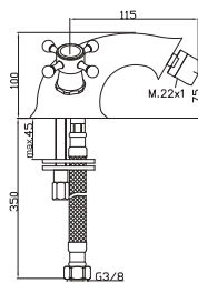
Bidet mixer
