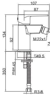
Bidet mixer
