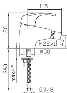
Bidet mixer
