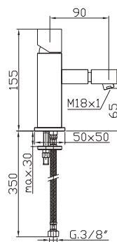
Bidet mixer
