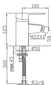
Bidet mixer
