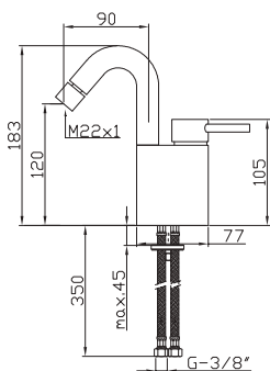
Bidet mixer
