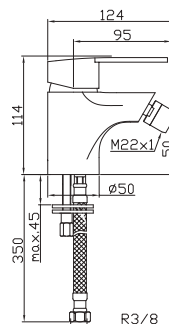
Bidet mixer
