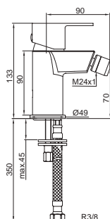
Bidet mixer
