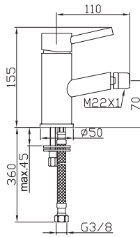
Bidet mixer
