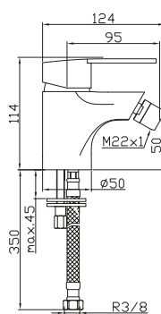
Bidet mixer
