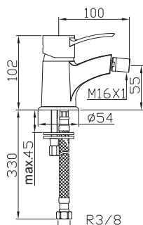
Bidet mixer
