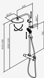
Columna Telescópica
