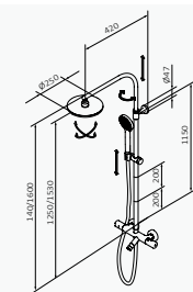
Columna Telescópica
