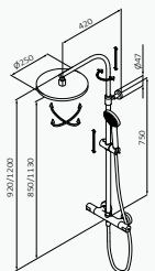
Columna Telescópica
