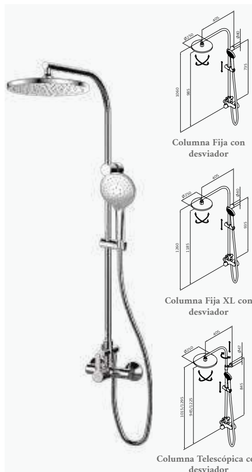
Columna Telescópica
