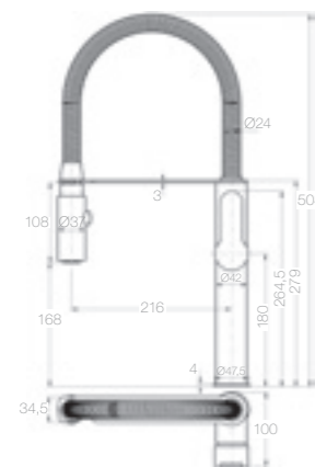
F9 MONOMANDO FREGADERA CON MUELLE EXTRAÍBLE REF. 65809
