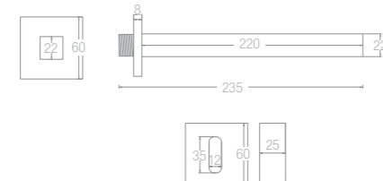
STAR SQUARE GRIFO EMPOTRADO ELECTRÓNICO REF. 14018 / 14017
