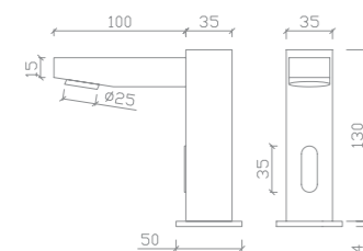
STAR SQUARE GRIFO ELECTRÓNICO LAVABO REF. 14028 / 14027
