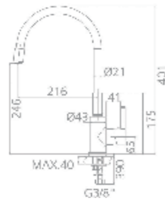
F18 MONOMANDO FREGADERA FLEXIBLE NEGRO REF. 65818
