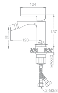
MONOMANDO BIDÉ REF. 68132 / 68132-Sline
