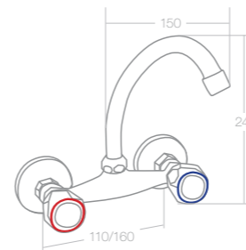
BATERÍA FREGADERA CAÑO VERTICAL REF. 65905 / 65904
