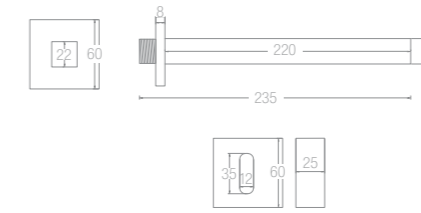
STAR SQUARE GRIFO EMPOTRADO ELECTRÓNICO REF. 14018 / 14017
