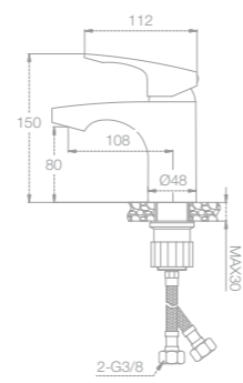
MONOMANDO LAVABO REF. 68161 / 68161-Sline
