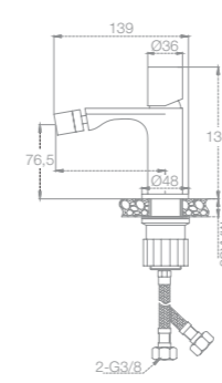
MONOMANDO BIDÉ REF. 68192 / 68192-Sline
