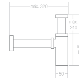
SIFÓN LUX / LATÓN-CROMO REF. CA-41430
