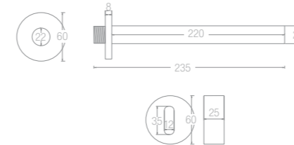
STAR ROUND GRIFO EMPOTRADO ELECTRÓNICO LAVABO REF. 14016 / 14015
