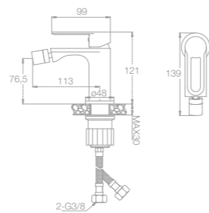
MONOMANDO BIDÉ REF. 68152 / 68152-Sline
