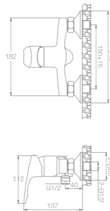
MONOMANDO DUCHA REF. 68164 / 68164-Sline
