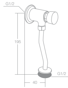
GRIFO TEMPORIZADO URINARIO FRONTAL REF. 14035
