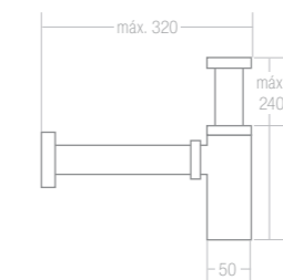
SIFÓN BOTELLA CROMADO REF. CA-41432
