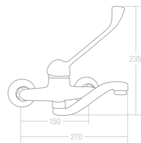
MONOMANDO FREGADERA PARED (CAÑO BAJO) REF. 14054
