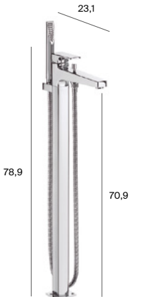
Columna monomando de pie para baño-ducha
