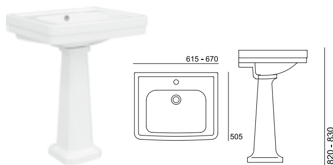
Lavatório . Lavabo . Washbasin 16321XX2C [67x50x23cm] 16331XX2C [61x50x23cm]
