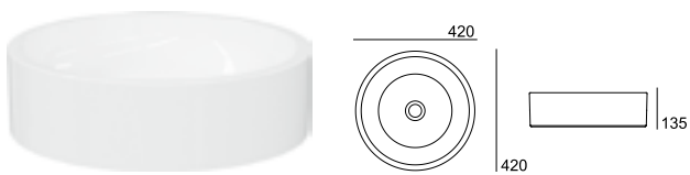
Malibu Lavatório . Lavabo . Washbasin 78737XX2C
